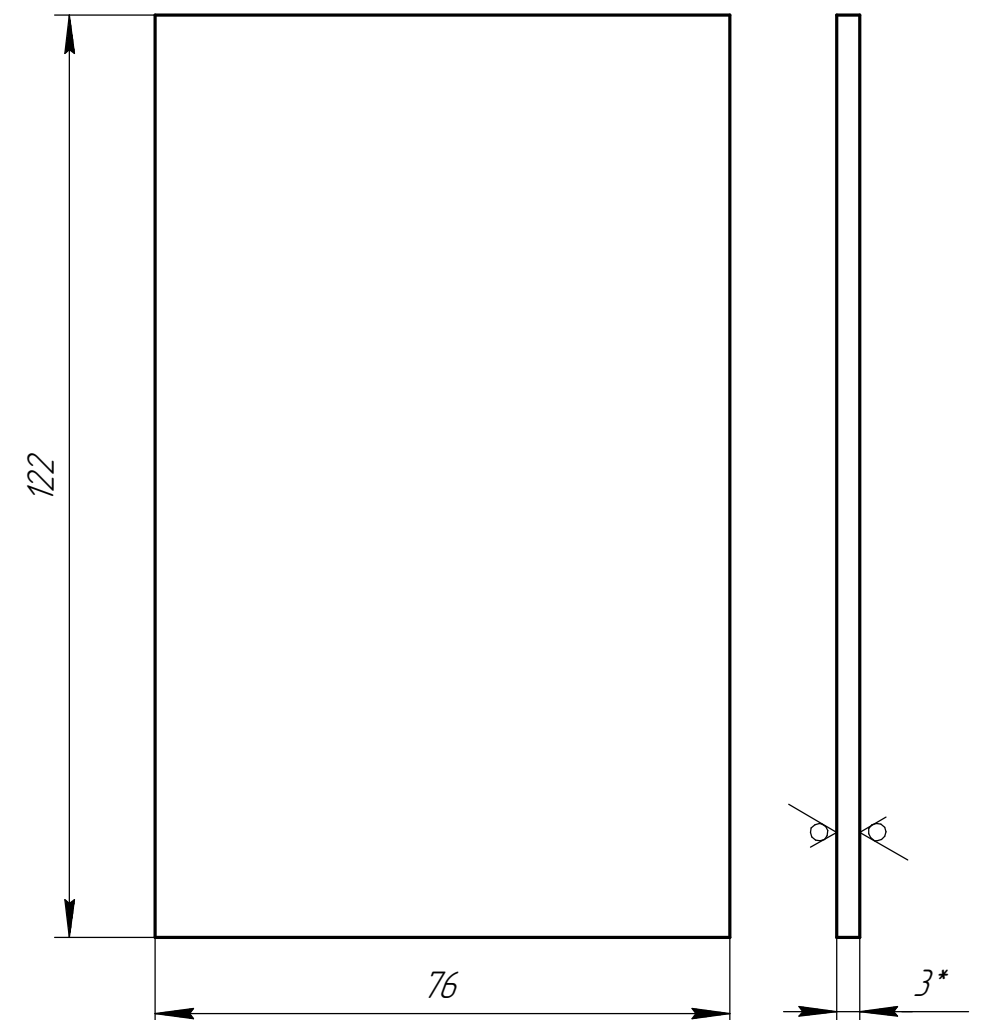
Дет. поз. 1
