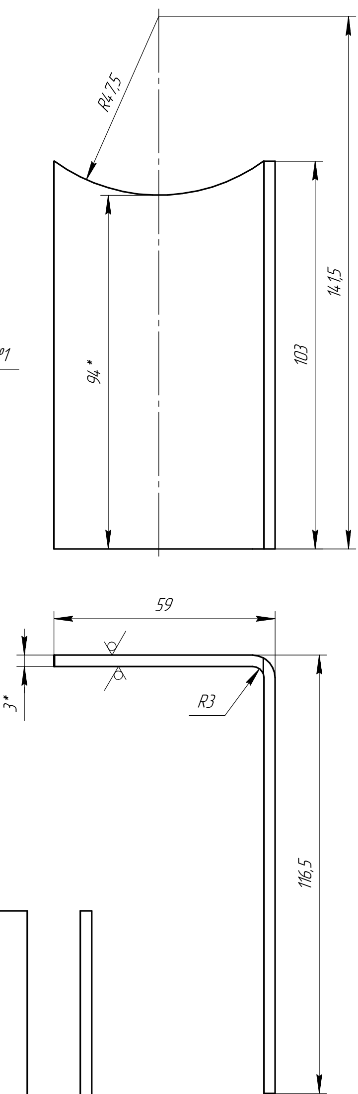
Дет. поз. 2
