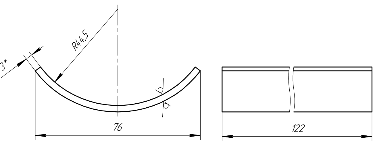
Дет. поз. 3
